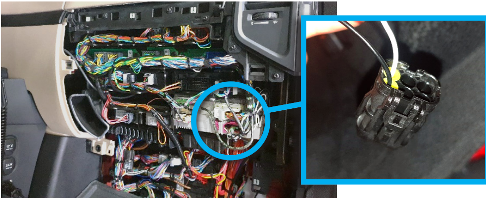
CAN 신호 커넥터 형상 및 핀 배열
