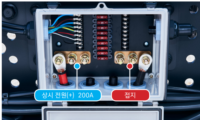
특장용 정선 박스 내부 배터리 단자
