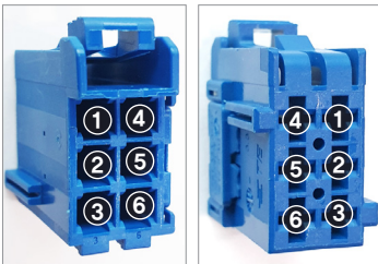
전원 커넥터 형상 및 핀 배열
